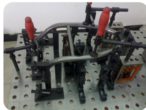
三维柔性焊接工装
